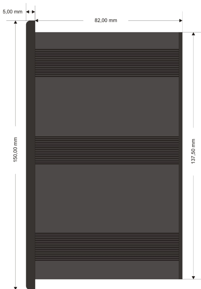
俯视图
